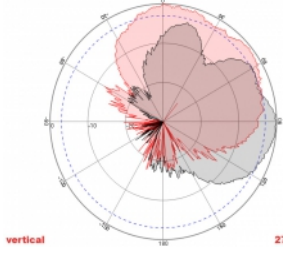
vertical 2700MHz
