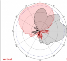
vertical 2500MHz
